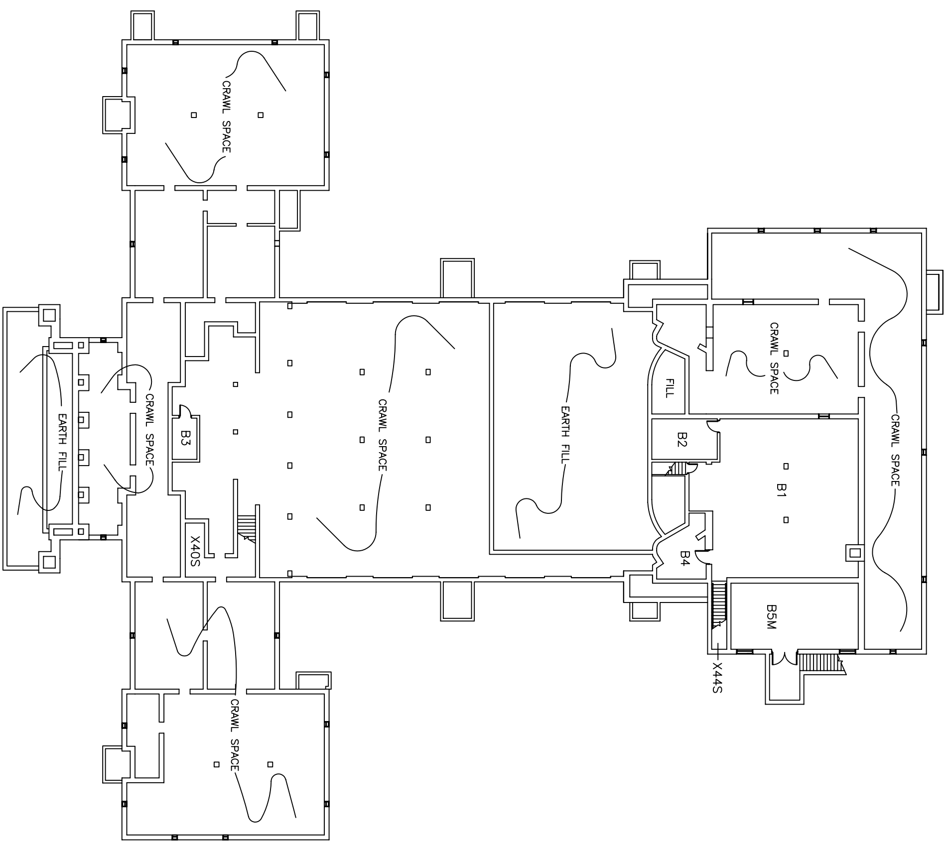
1 A1.1 SCALE: 3/32"=1'-0"
